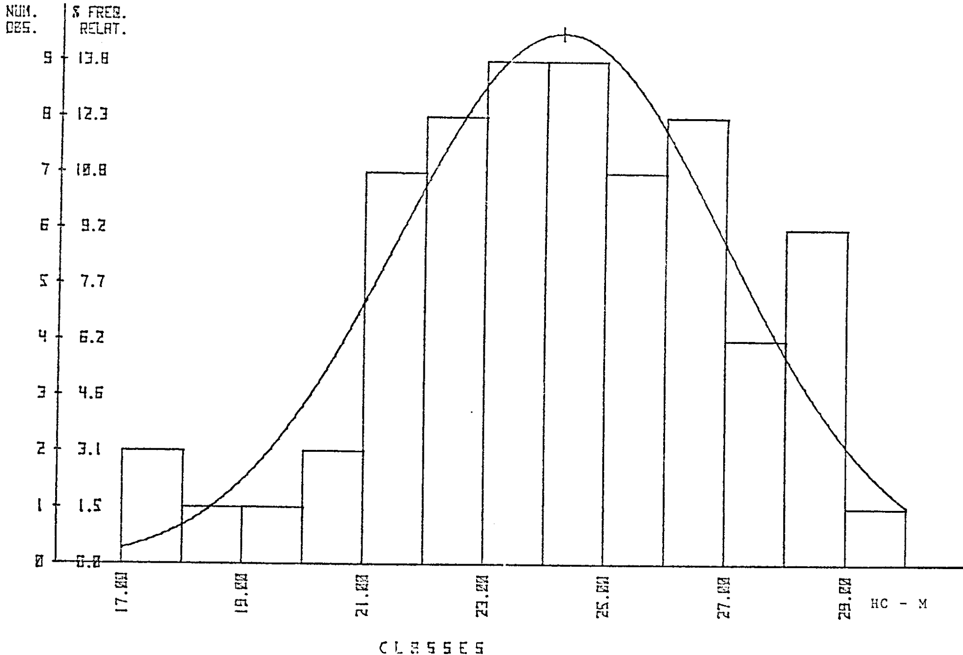
FIGURA 6 - Histograma médio relativo à distribuição porcentual de freqüências relativas por classes de altura comercial, para as posições correspondentes ao 3º ponto de interseção
