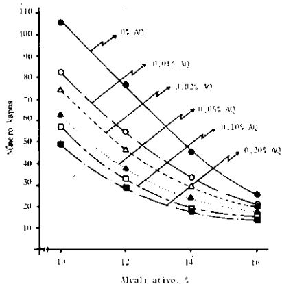
FIGURA 4 - Relação entre número kappa e álcali ativo, em cozimentos soda, com adição de diferentes dosagens de antraquinona.
