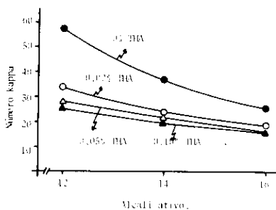
FIGURA 13 - Relação entre número kappa e álcali ativo, em cozimentos soda, com adição de diferentes concentrações de tetraidroantraquinona.
