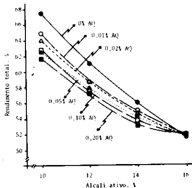
FIGURA 6 - Relação entre rendimento total e álcali ativo em cozimentos soda, com adição de diferentes dosagens de antraquinona.
