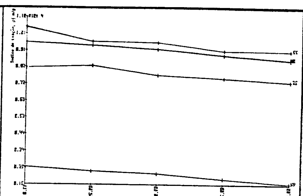
FIGURA 6 - Índice de tração nos níveis de refino estabelecidos em função da porcentagem de madeira de Acácia mangium na mistura.
