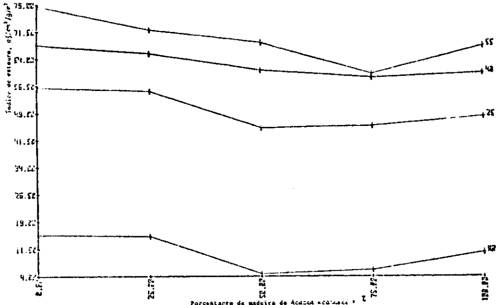
FIGURA 9 - Índice de escurecimento nos níveis de refino estabelecidos em função da porcentagem de madeira de Acacia mearnsii na mistura
